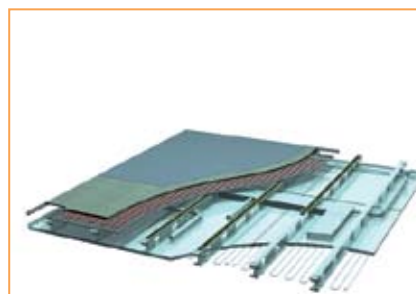
TOPVLOER
