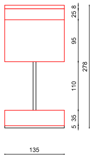
vooraanzicht
