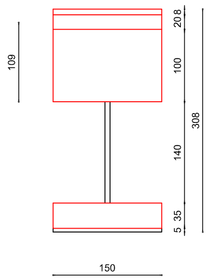
vooraanzicht
