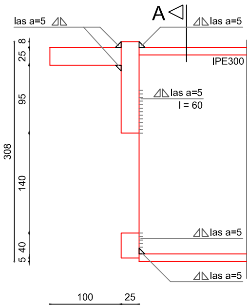
zijaanzicht
