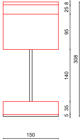
vooraanzicht
