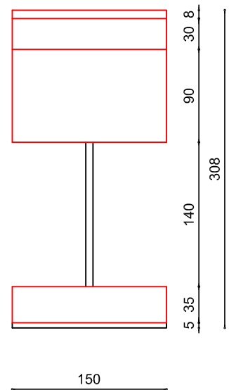
vooraanzicht
