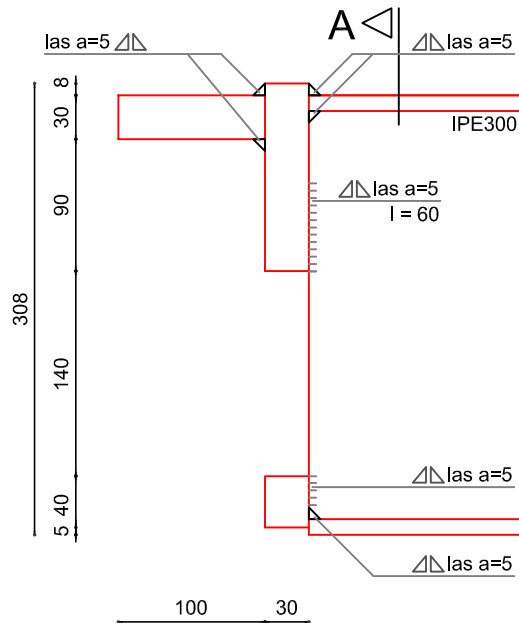
zijaanzicht
